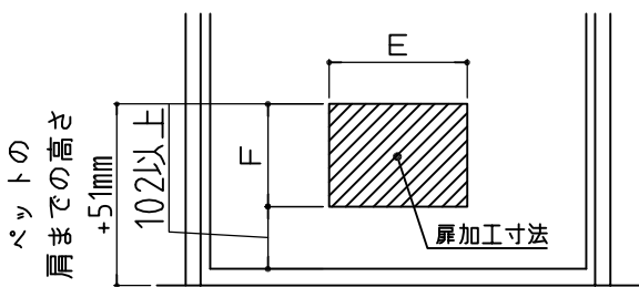
扉加工図
