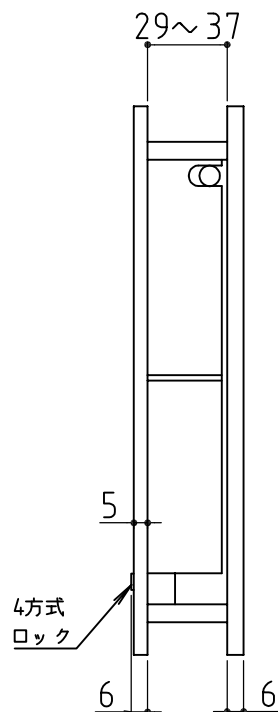
組込図
